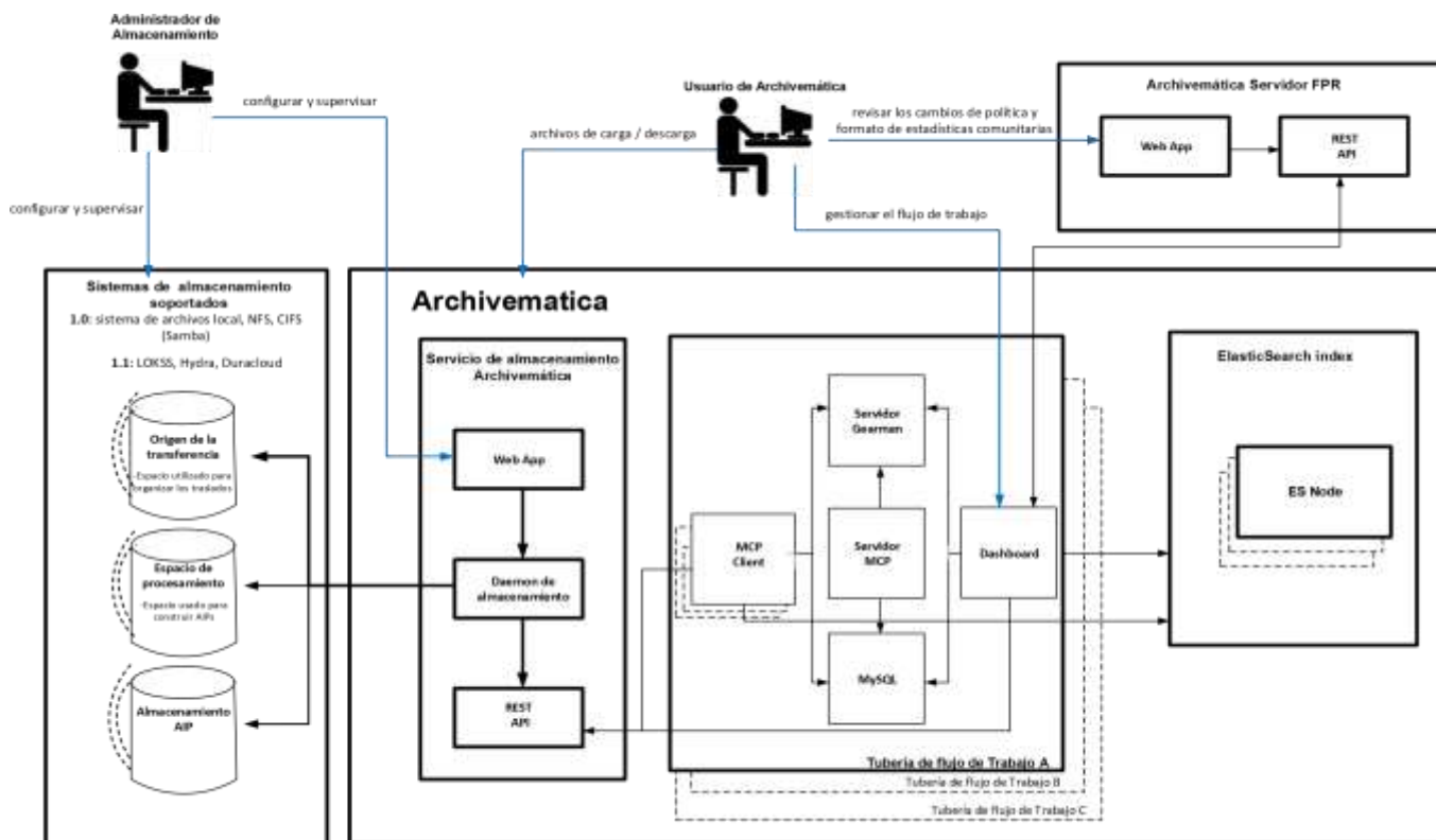
Figura 1: Diagrama de la arquitectura de Archivemática. Adaptado de (Artefactual, 2016).
